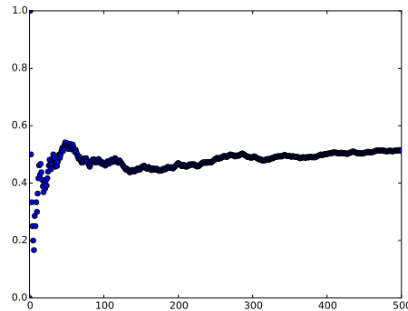
Figure 8: Traçage du graphe n \mapsto p_n , avec p_n proportion à l'instant n du nb de piles dans une suite de pile-face aléatoires indépendants, avec proba de pile valant 1/2 . On perçoit sur le dessin la convergence annoncée.
