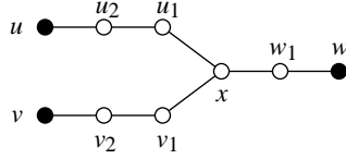
Fig. 10. Configuration of Lemma 31(3).
