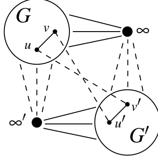
Fig. 3. The (0,2) -mixed tromp graph Tr(G) .
