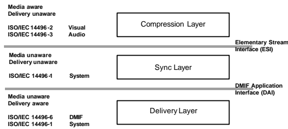
Fig. 1. MPEG-4 Framework
