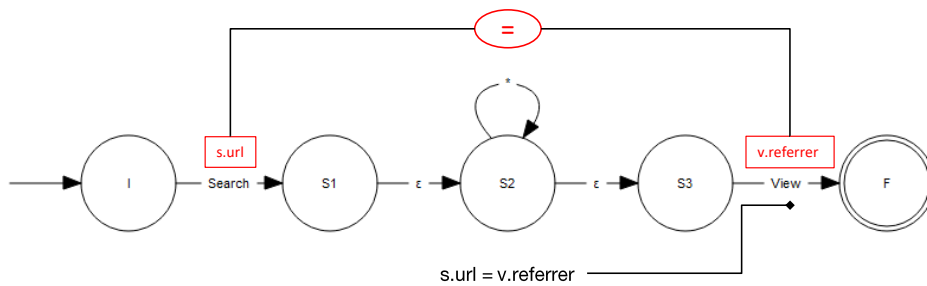
FIGURE 4.7 – Automate généré pour la règle SearchThenView. La transition de type View comporte un prédicat permettant de lier les événements s et v . Ce prédicat de lien permet de vérifier l'égalité entre les attributs url de l'évènement s , et referrer de l'évènement v .
