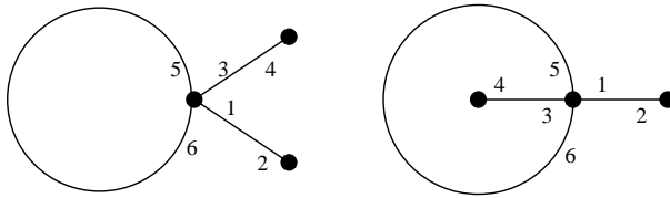
FIG. 6 – Exemple de codage de cartes par permutations
