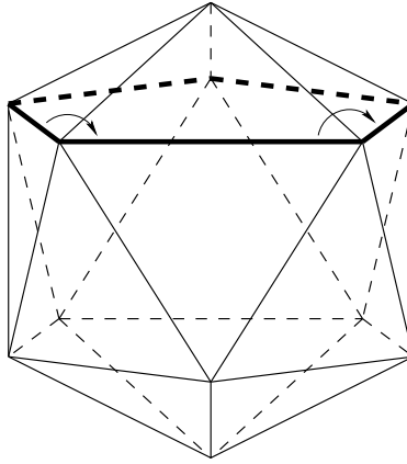
FIG. 8 – Un cycle de longueur 5 de la permutation \alpha^{-1}\sigma^{-2}
