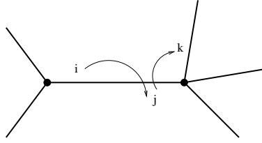
FIG. 7 – Comment « calculer » les faces d’une carte en connaissant les permutations \sigma et \alpha : pour aller autour d’une face dans le sens trigonométrique il faut répéter les permutations \alpha^{-1} et \sigma^{-1}
