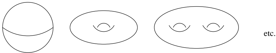
FIG. 2 – Les variétés compactes orientables de dimension 2 et de genre g = 0 (la sphère), g = 1 (le tore) et g = 2 .
