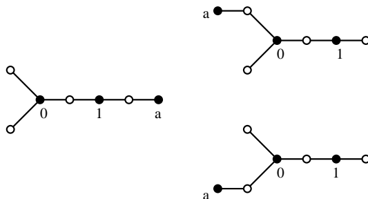
FIG. 11 – Une orbite cubique de l'action du groupe de Galois ; le corps de nombres associé à cette orbite est l'extension de \mathbb{Q} par les racines cubiques de 2
