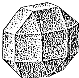
FIG. 13 – Le pseudorhombicuboctaèdre
