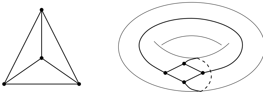
FIG. 5 – Le graphe complet K_4 dessiné sur la sphère et sur le tore
