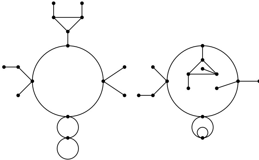
FIG. 4 – Le même graphe mais des cartes différentes
