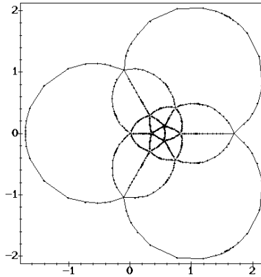
FIG. 12 – Le « dessin d'enfant » de l'icosaèdre
