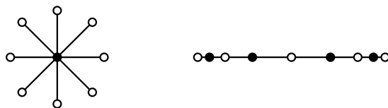
FIG. 10 – L'arbre-étoile et l'arbre-chaîne
