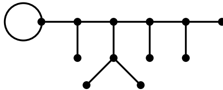
FIG. 9 – Une carte représentant le groupe de Mathieu M_{24} : elle possède 12 arêtes, donc 24 brins ; les permutations \sigma et \alpha correspondantes agissent sur 24 éléments et engendrent le groupe M_{24}
