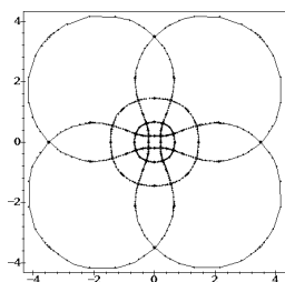
FIG. 14 – Le « dessin d'enfant » du pseudorhombicuboctaèdre
