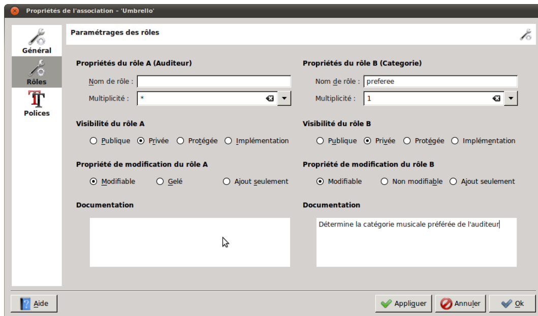
FIGURE 4 – édition des propriétés d’une association.
