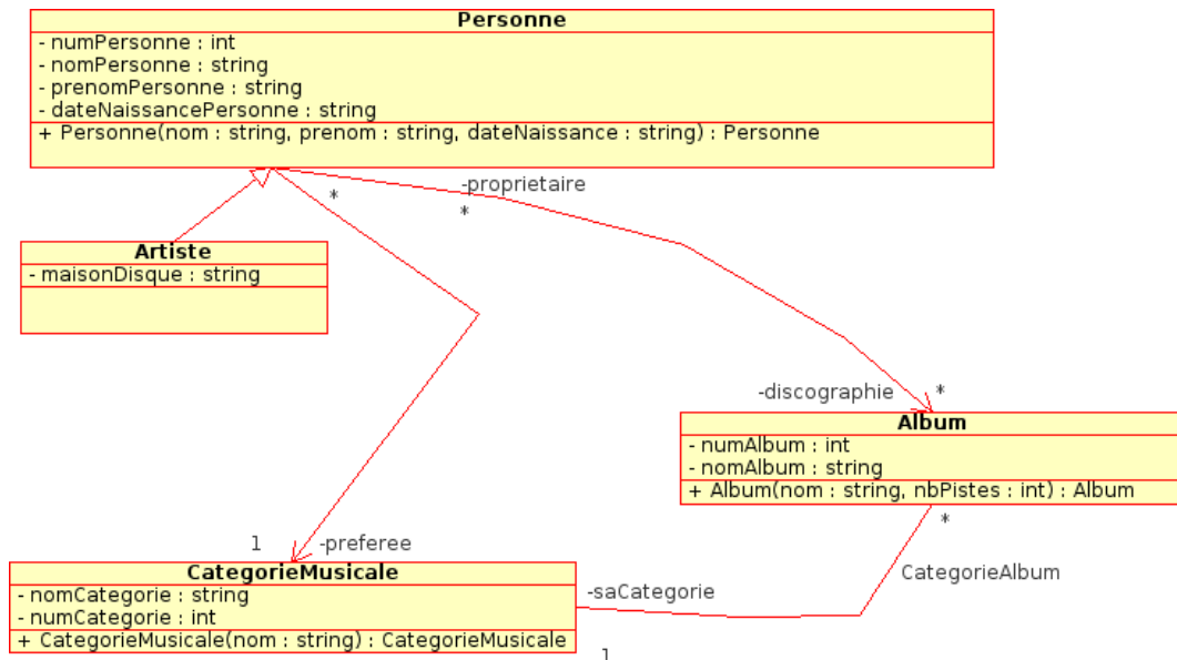
FIGURE 1 – Une solution au sujet d'exemple.
