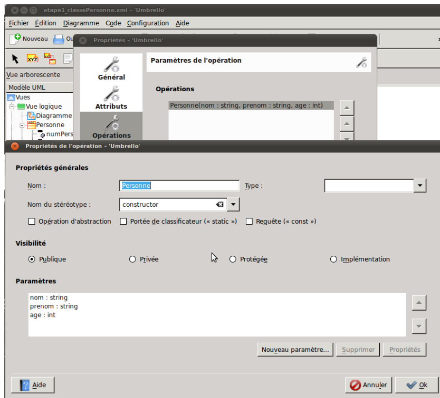
FIGURE 3 – Propriétés de la classe Personne et édition du constructeur paramétré.
