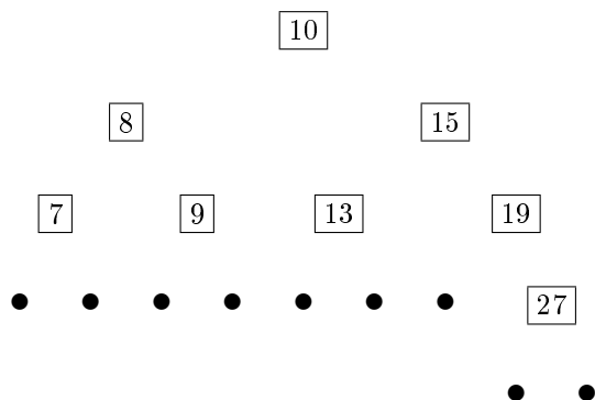
FIG. 12.1 – Un arbre binaire de recherche
