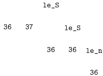
FIG. 5.1 – Une preuve de l’inégalité 36 \leq 38
