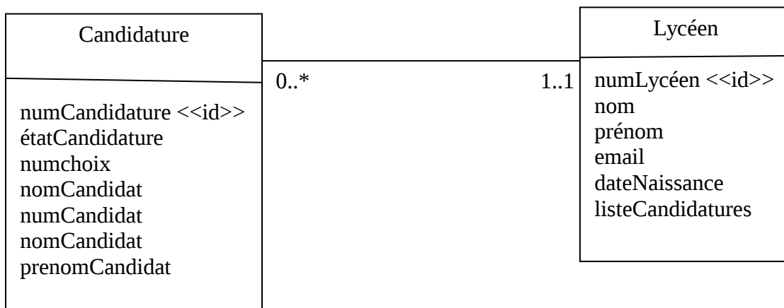
Diagramme de classes 3 :
