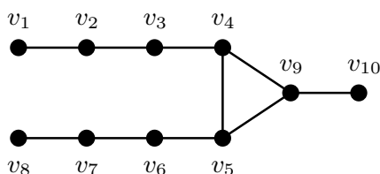
Figure 5 – Le troisième sous-graphe induit interdit.
