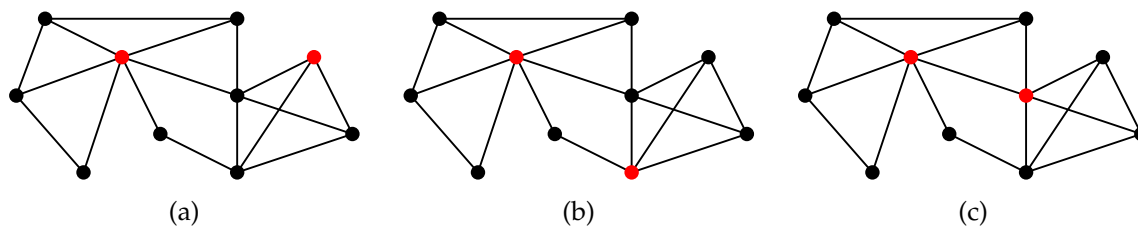
Figure 3 – Trois nouveaux ensembles dominants de taille deux du même graphe.
