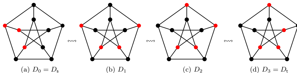
Figure 4 – Séquence de reconfiguration d'ensembles dominants du graphe de Petersen.
