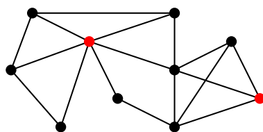
Figure 2 – Ensemble dominant minimum de taille deux d'un graphe.
