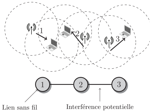
FIGURE 1. Un exemple de graphe d'interférence
