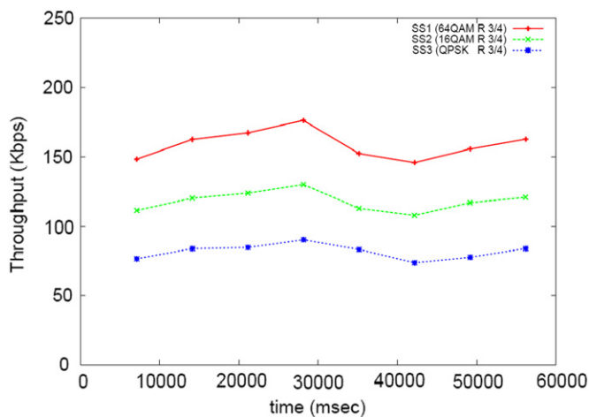
Fig. 23. Multiple coding scheme scenario.
