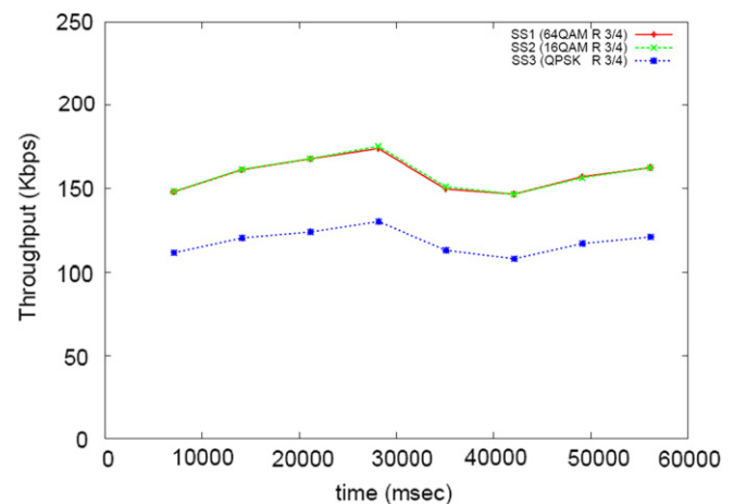
Fig. 24. Scenario: superposition coding scheme.
