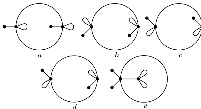
Рис. 1: Пять карт с паспортом (5^2 1^2, 2^6, 5^2 1^2) .
